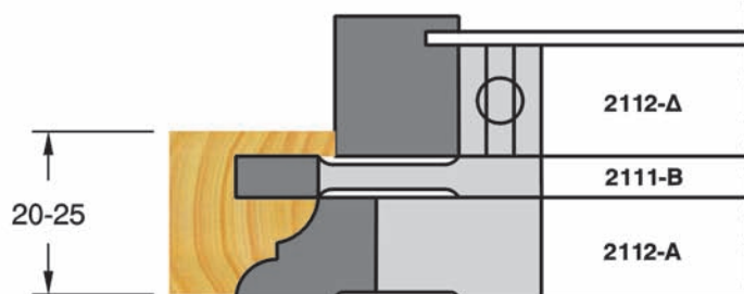
2112-2 με 2 εργαλεία & ροδέλλα
