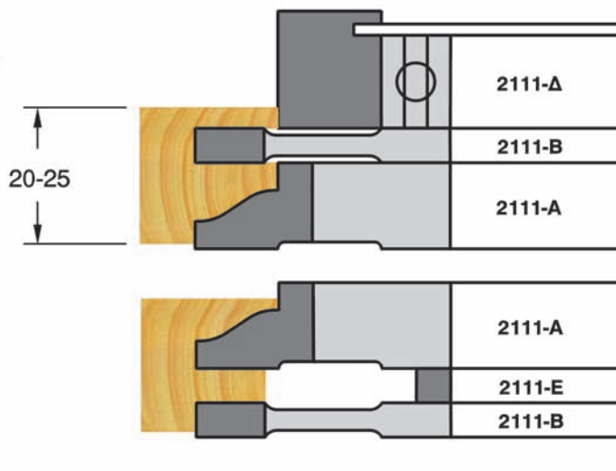
2111-2 με 2 εργαλεία & ροδέλα
